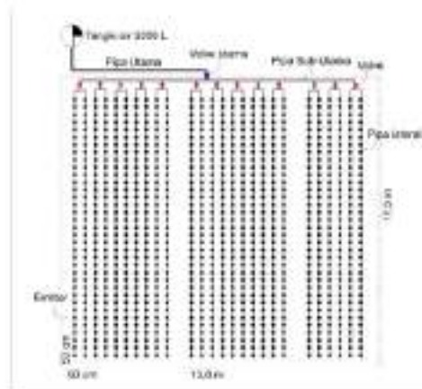
Gambar 1. Rancangan irigasi tetes di lahan pertanian cabai rawit Desa Slengen
