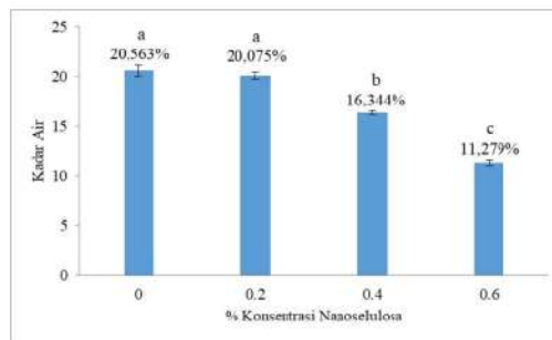
Gambar 1. Nilai Kadar Air Bioplastik
