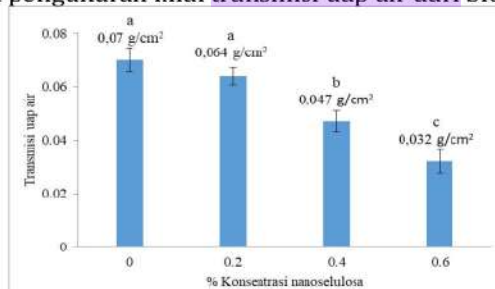
Gambar 4. Nilai Transmisi Uap Air Bioplastik
