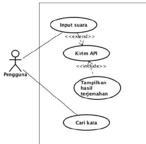
Gambar 3. Use Case Diagram Sistem yang Dibangun
