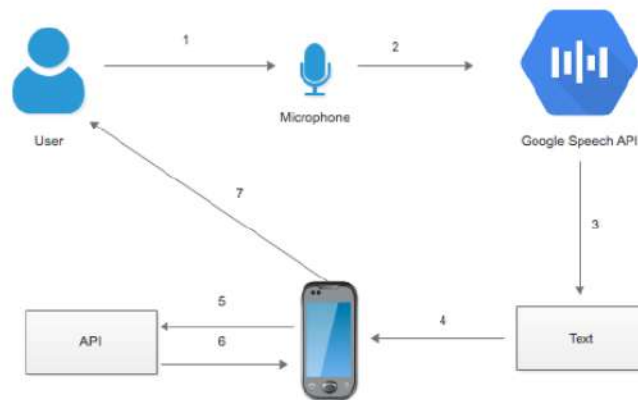
Gambar 2. Arsitektur Sistem yang Dibangun
