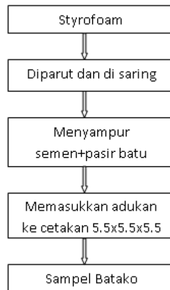
Gambar 1. Diagram alir pembuatan Batako
