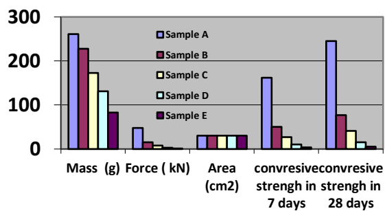
Gambar 4. Grafik Uji Karakteristik Batako Styrofoam
